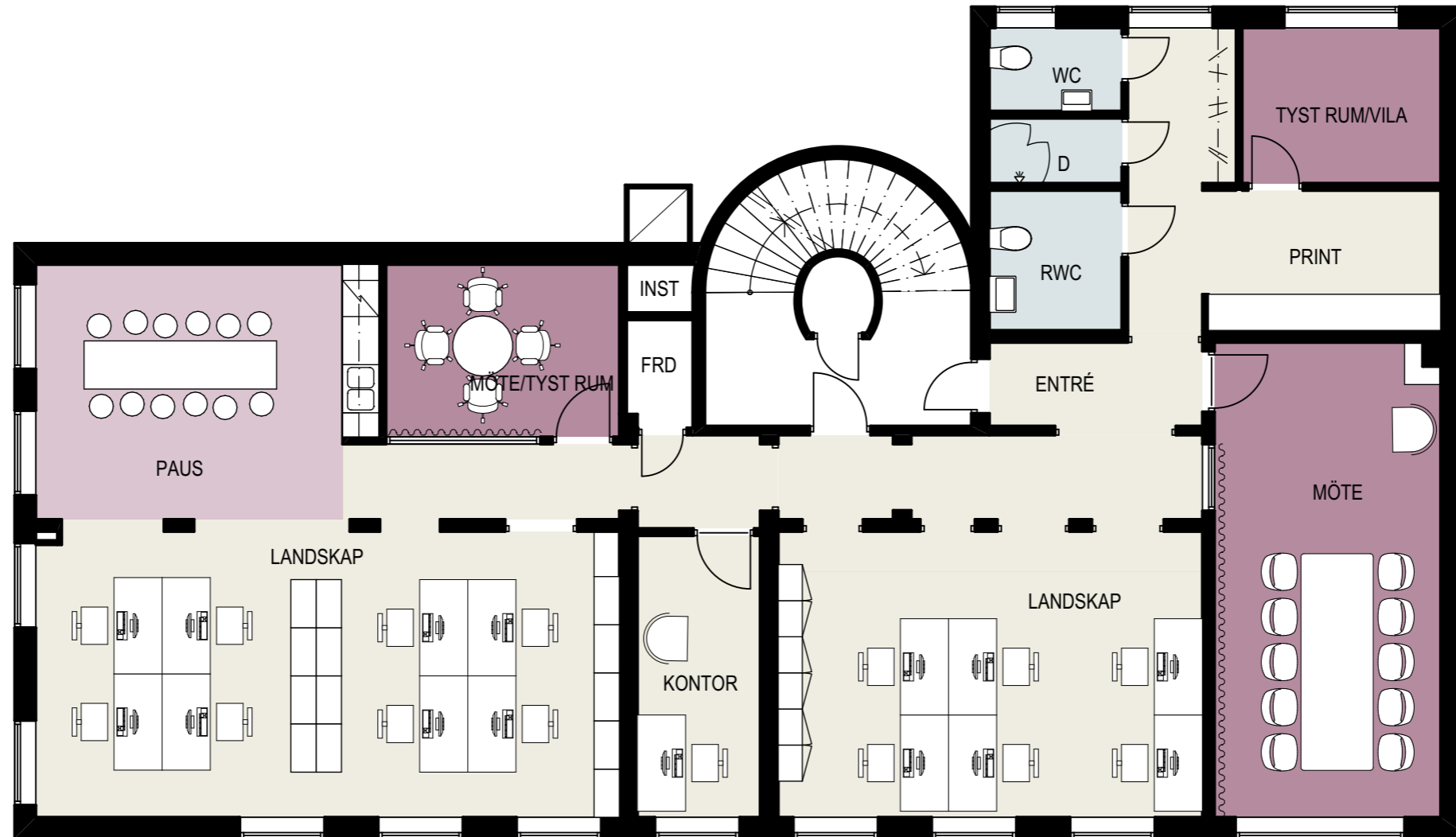
PLAN 2 1:100
