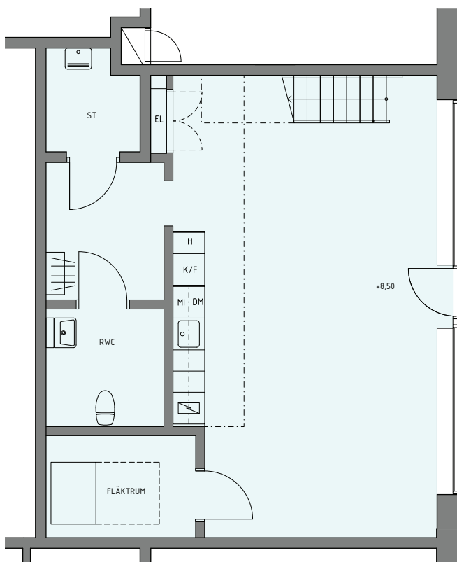
Plan 10, entréplan
