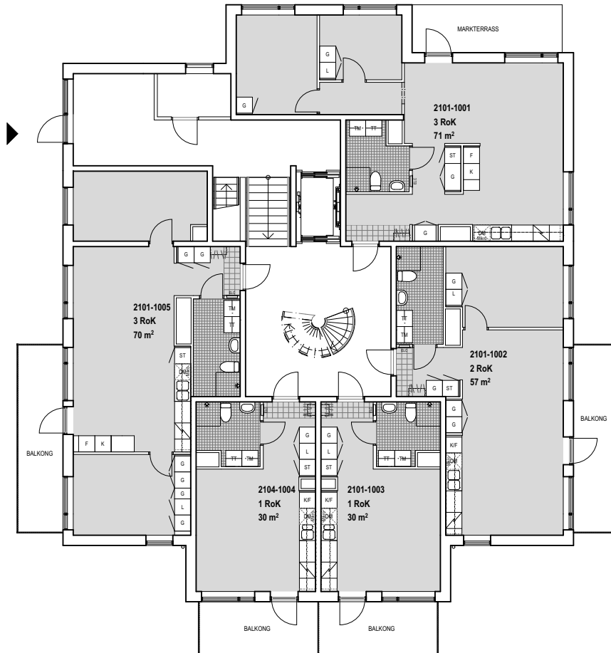
VÅNING 1
