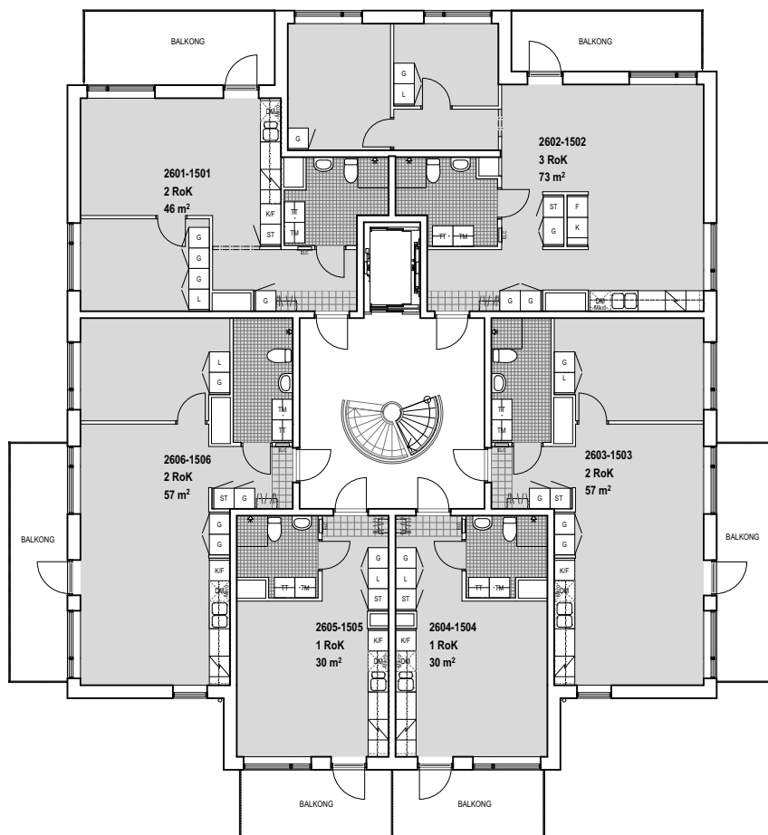
VÅNING 6
