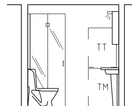
ELEVATION C SKALA 1:50
